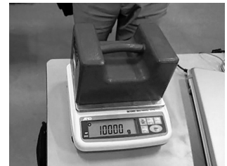
10kg標準分銅による補正
